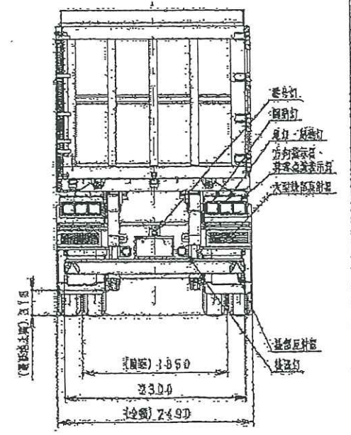
東邦TF36H2C3改型 ダンプセミトレーラ外觀四面図
